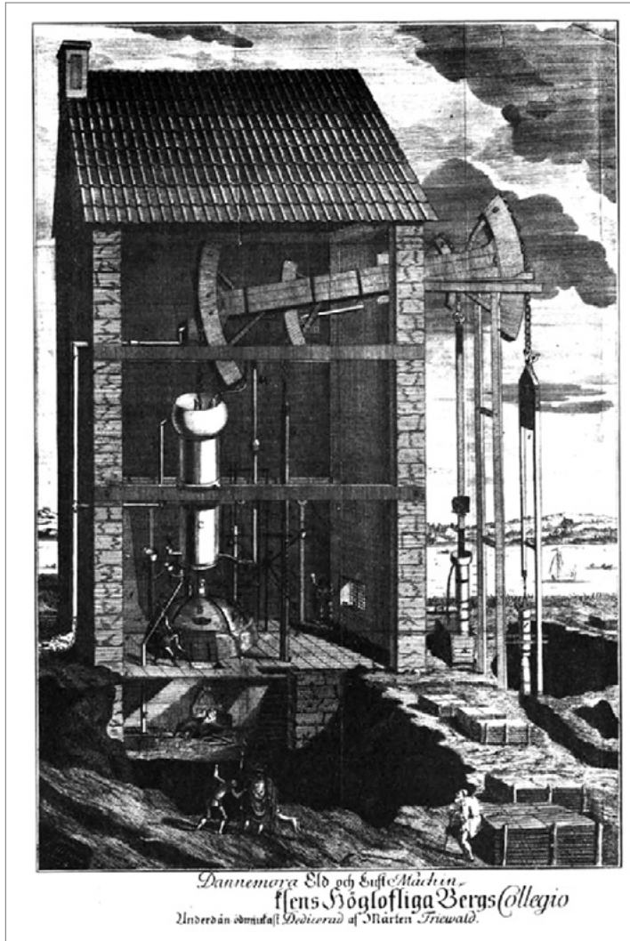
Φωτ.1. Γκραβούρα που απεικονίζει τη μηχανή του Νιουκάμεν, σε ορυχεία στη Ντανεμόρα, στη Σουηδία (Ferguson, 1963,99)
